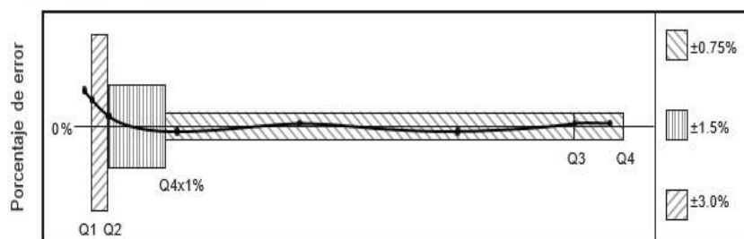
Curva típica de errores del Q4000
